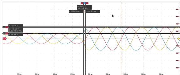
电压跌落波形
