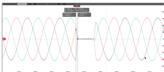
零电压穿越
